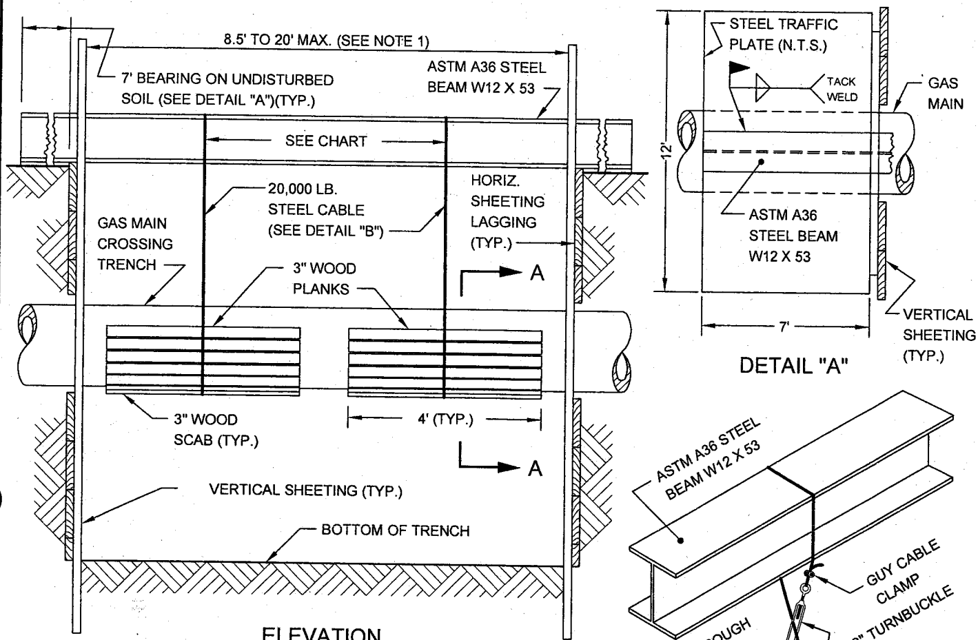
ELEVATION
