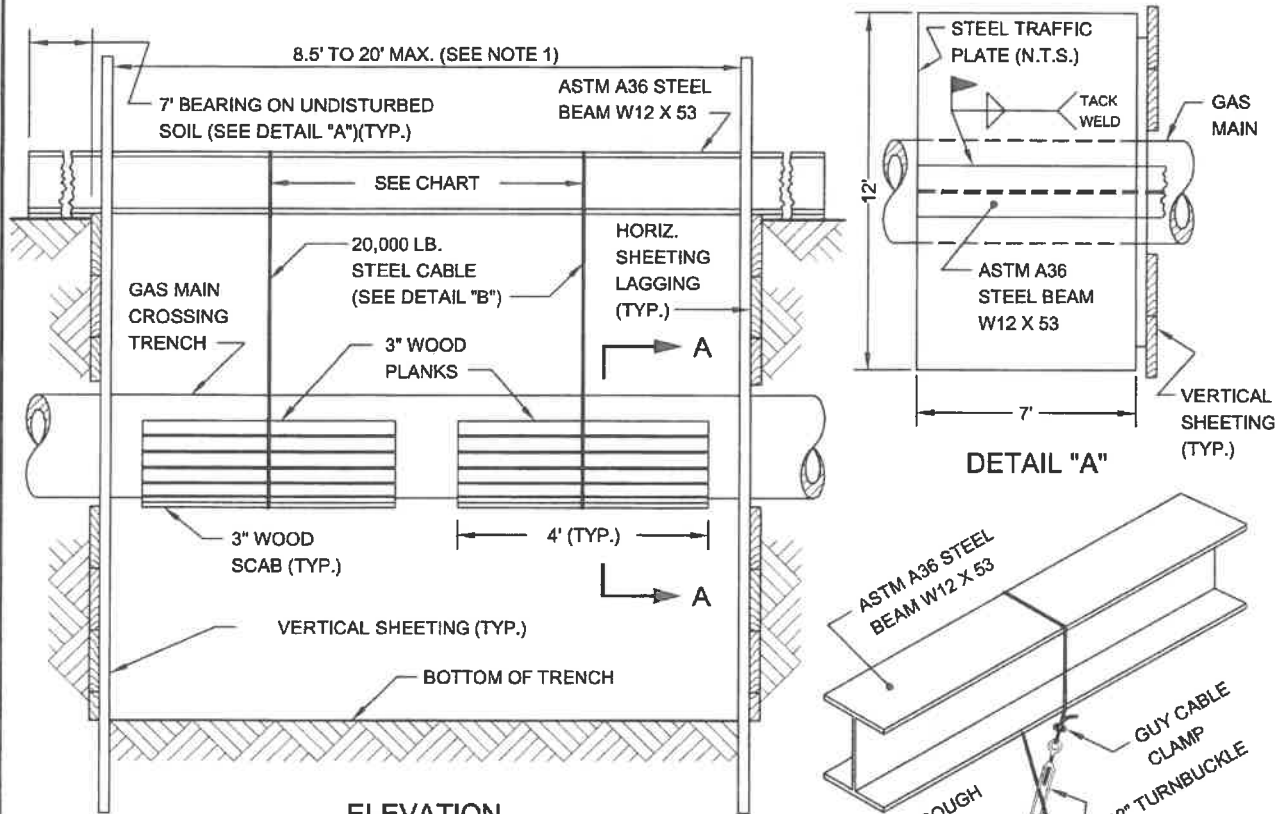
ELEVATION
