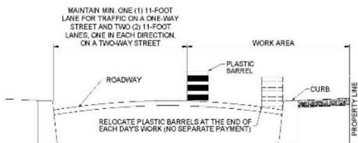
SECTION A-A 410
