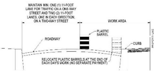
SECTION A-A 1/12
