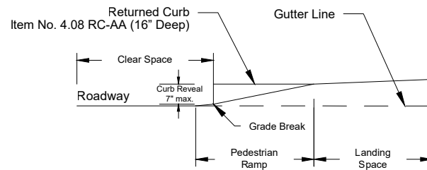
ELEVATION VIEW C-C (N.T.S.)
