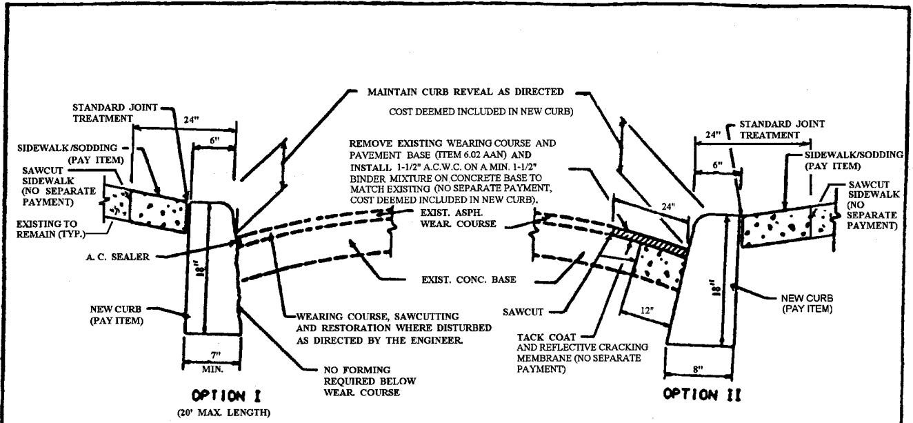
CURB RESTORATION DETAIL N. T. S.
