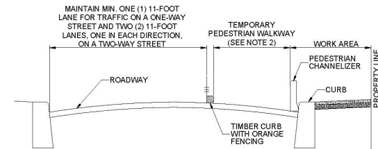
SECTION A-A 1/16
