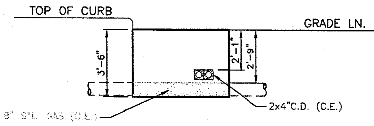
PROFILE - LOOKING WEST N.T.S.
