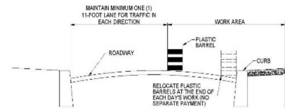
SECTION A-A 1/4\"/>
