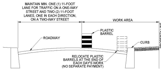
SECTION A-A N.T.S.
