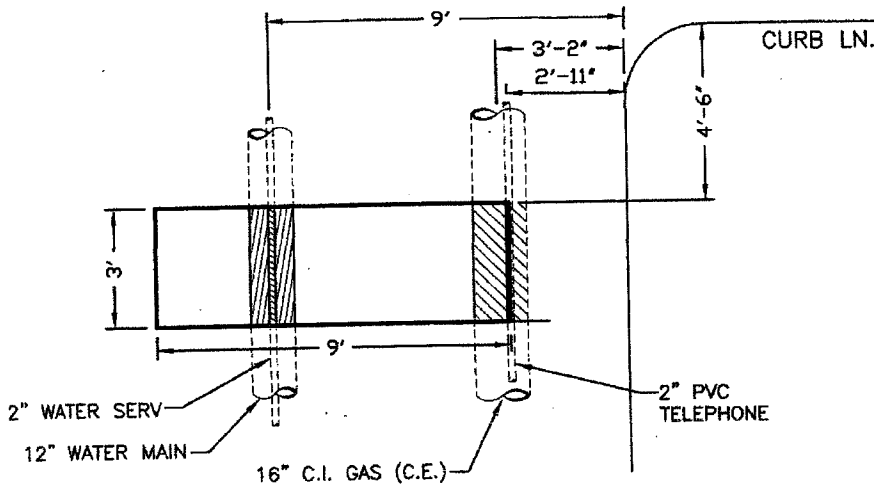
PLAN N.T.S.
