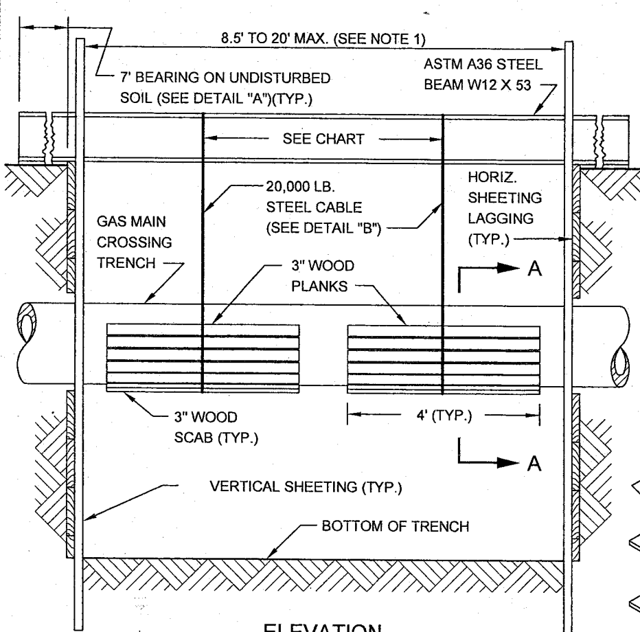
ELEVATION
