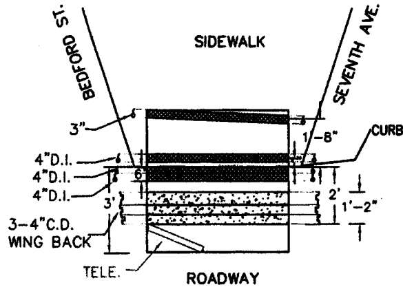
PLAN N.T.S.
