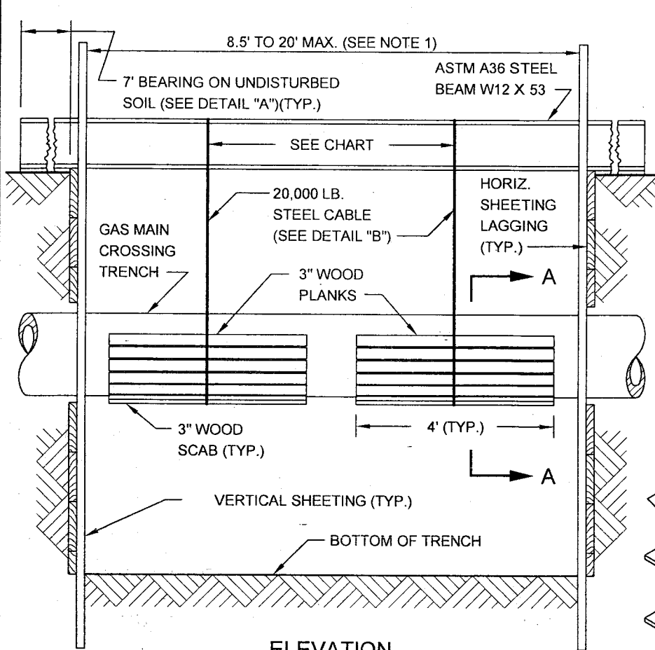
ELEVATION
