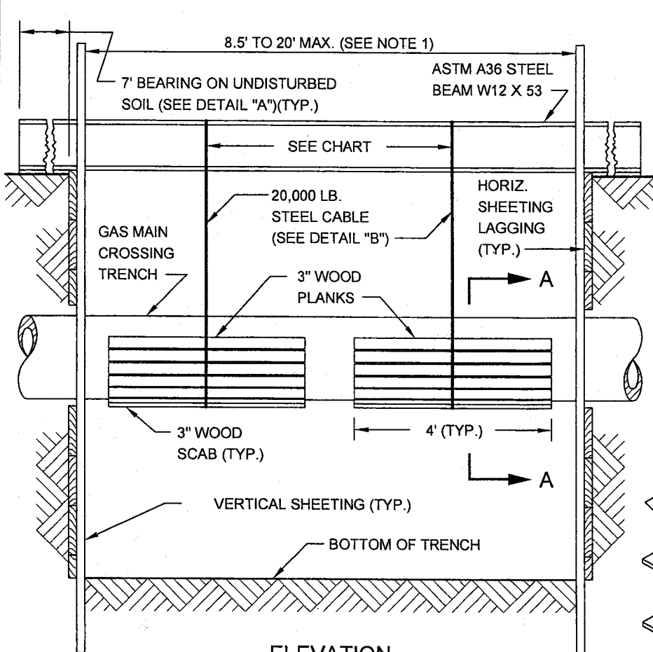
ELEVATION
