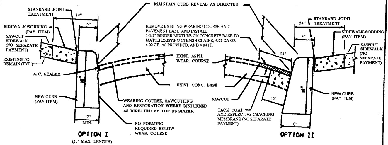
CURB RESTORATION DETAIL N. T. S.
